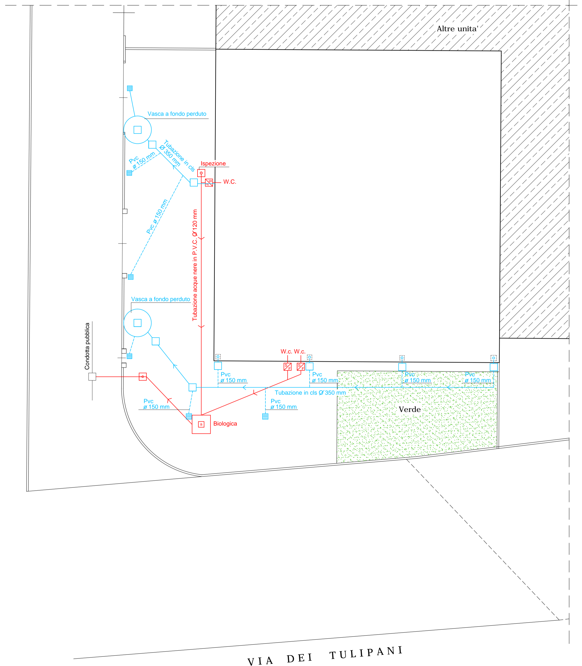
PLANIMETRIA RETE ACQUE NERE E METEORICHE SCALA 1:200
