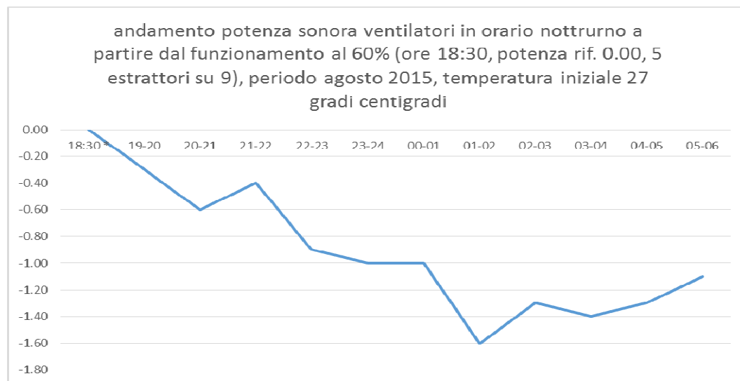
Grafico misura di repertorio ad illustrare il funzionamento notturno delle batterie di ventilatori.
