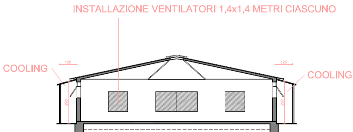
Dettaglio capannoni, sezione– Stato di progetto - non in scala – fonte: tavole di progetto
