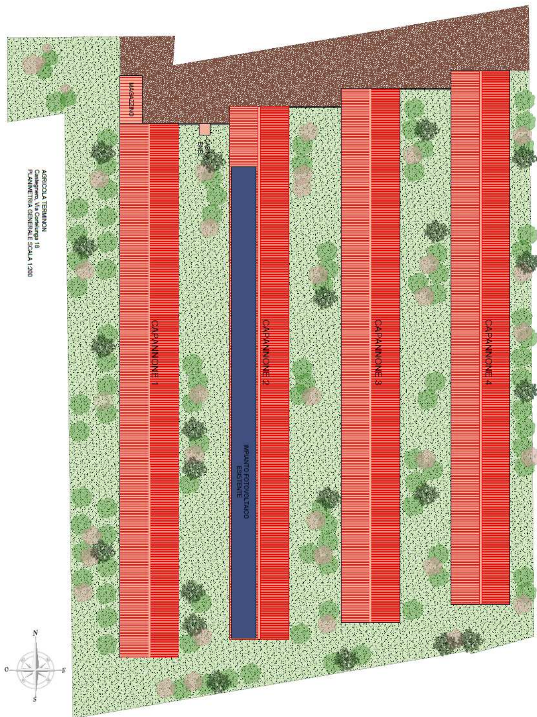
Planimetria allevamento – Stato di progetto - non in scala – fonte: tavole di progetto
