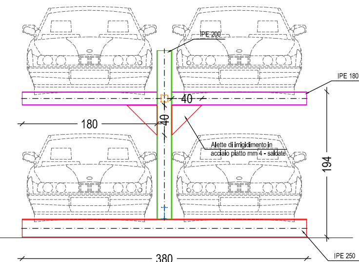
PROSPETTO LATERALE
