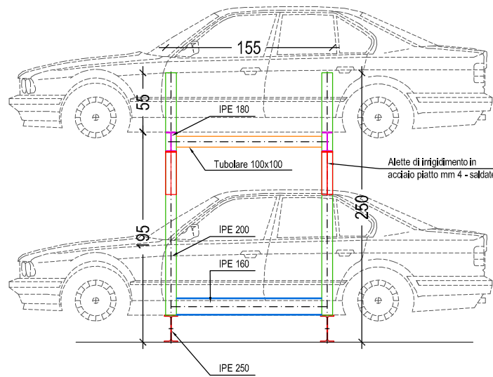
PROSPETTO FRONTALE
