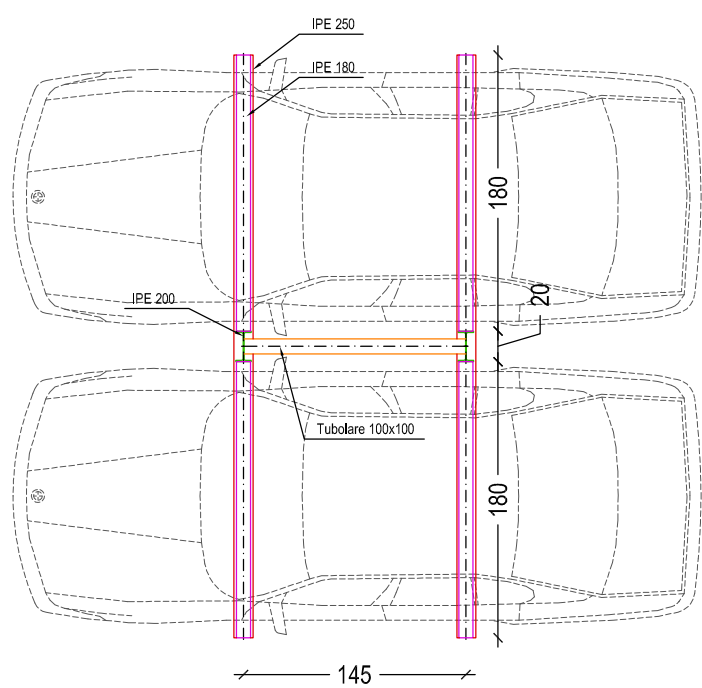
PIANTA
