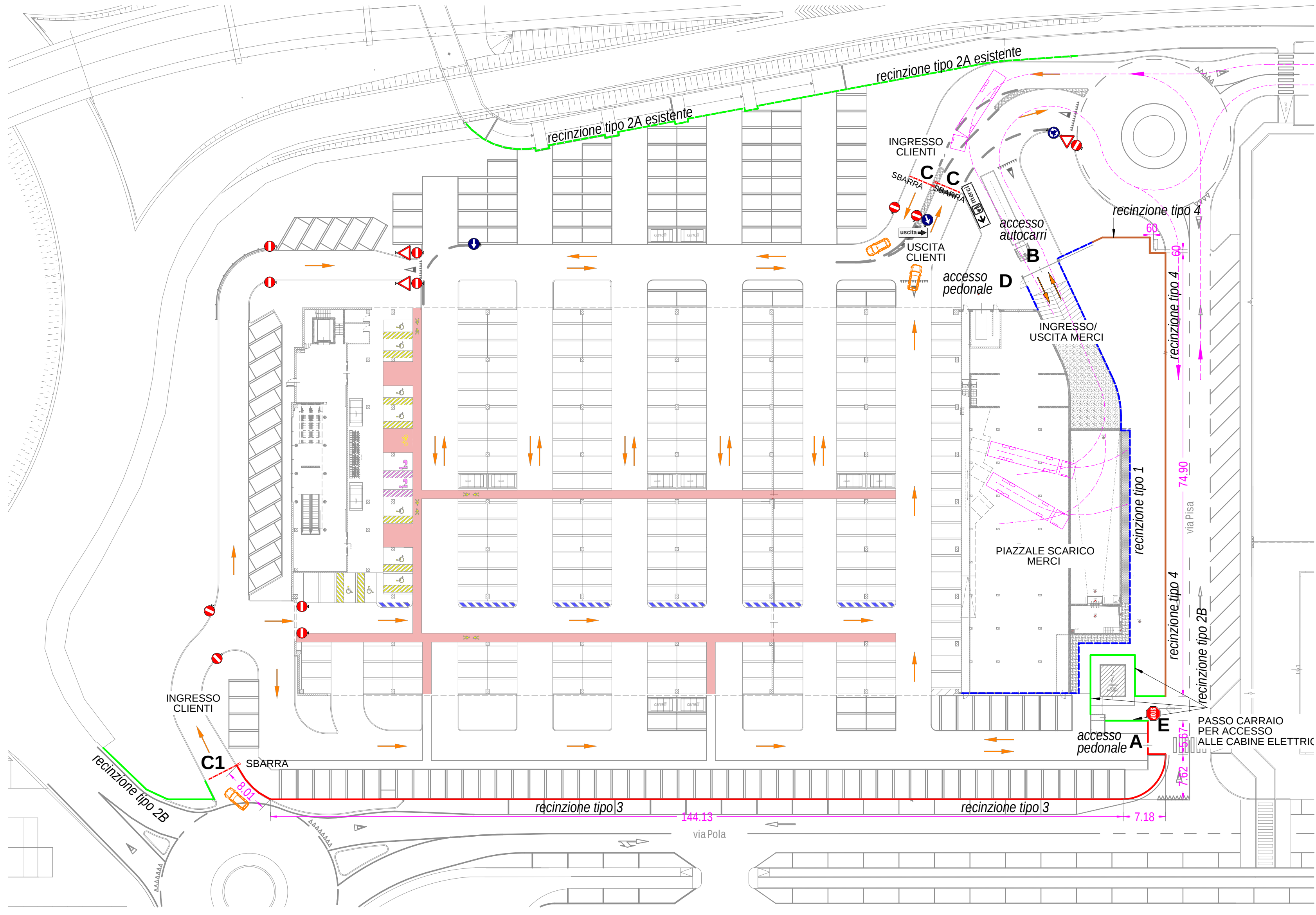
PLANIMETRIA CON INDICAZIONE DELLE RECINZIONI E DELLA VIABILITA' scala 1:500
