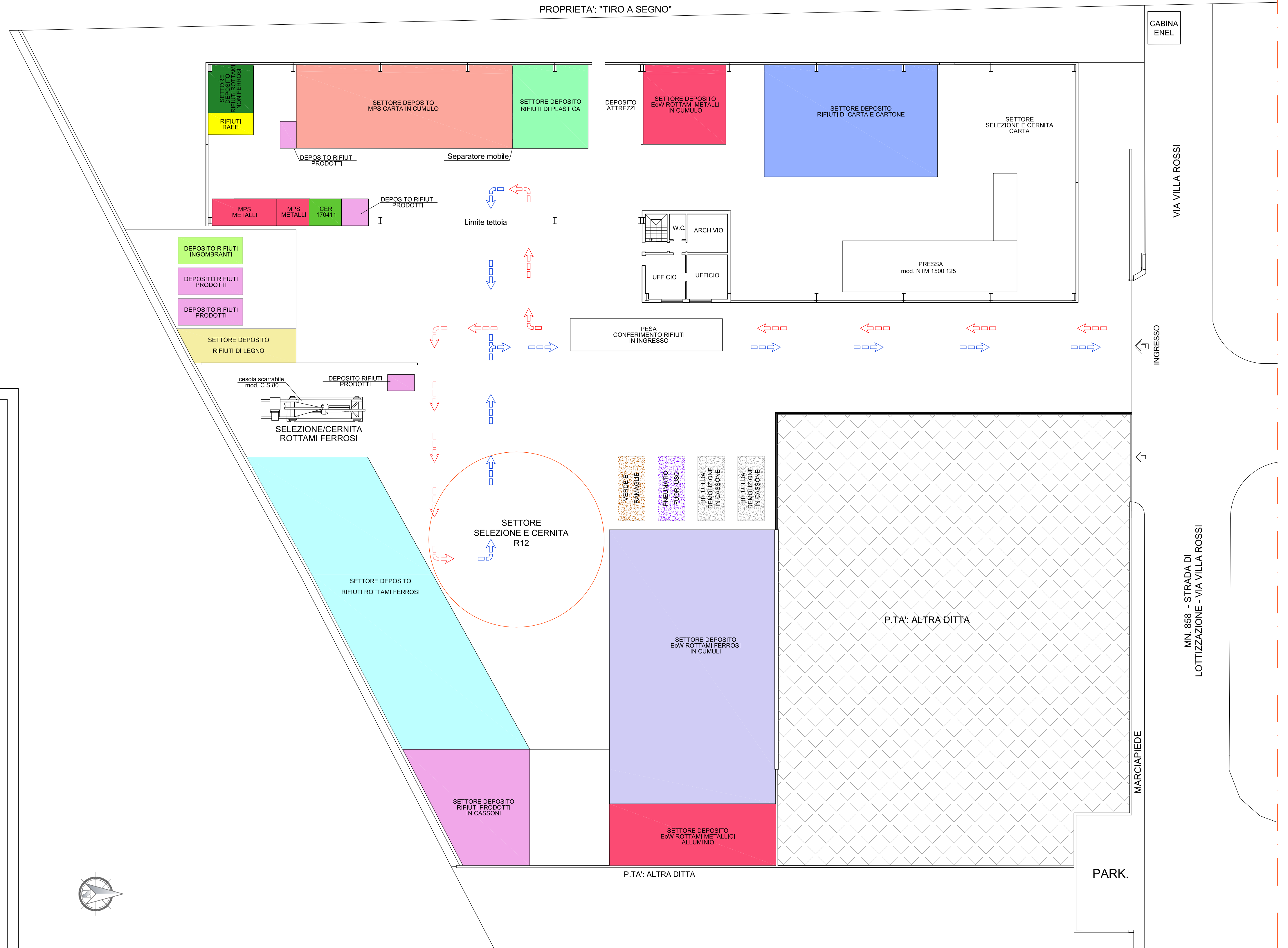
PLANIMETRIA GENERALE DI STATO DI PROGETTO SCALA 1:200
