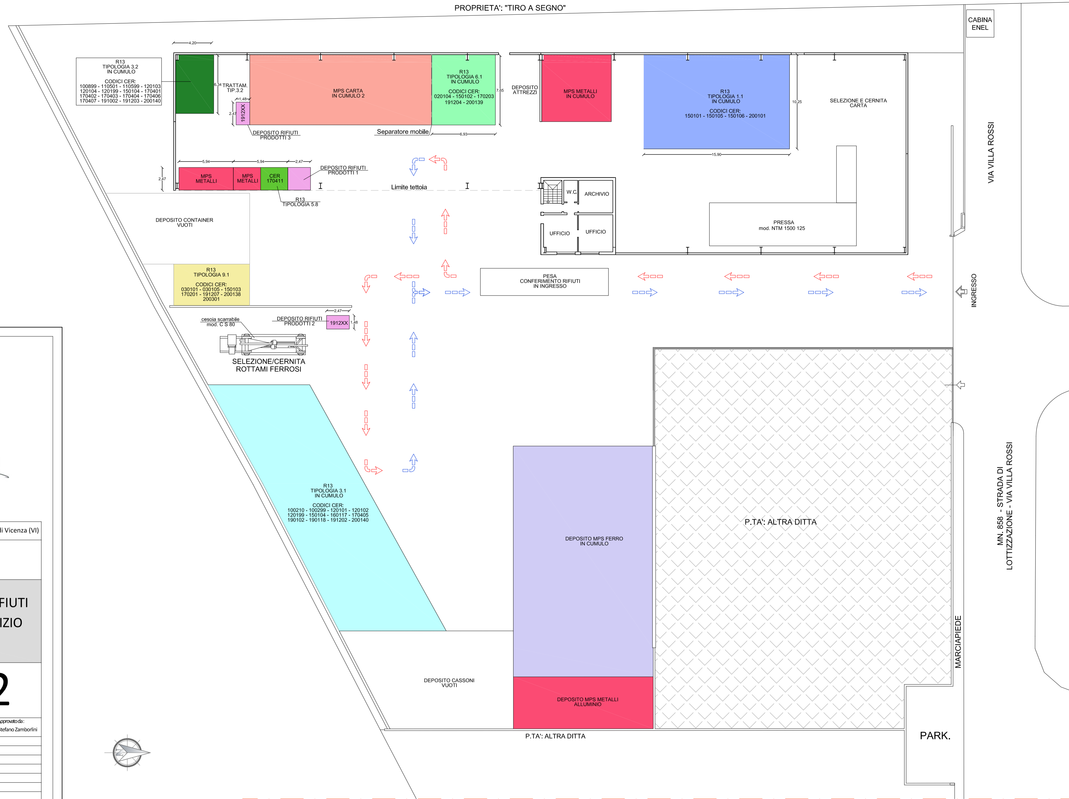
PLANIMETRIA GENERALE DI STATO DI FATTO SCALA 1:200
