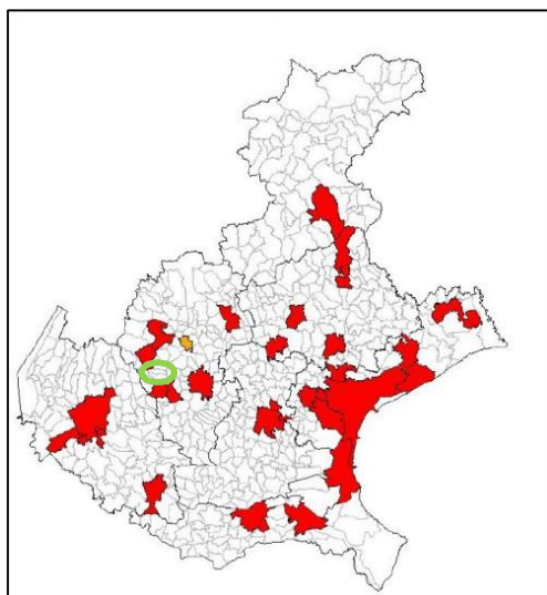
Monitoraggio IPA
