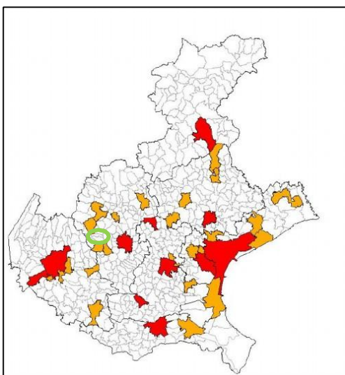
Monitoraggio NO 2
