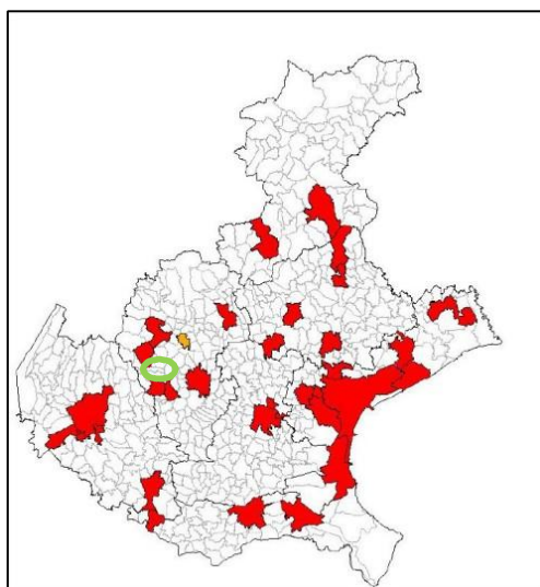
Monitoraggio PM10
