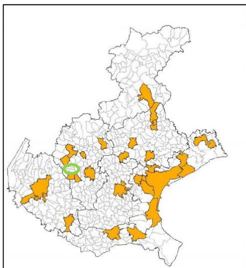
Monitoraggio BENZENE
