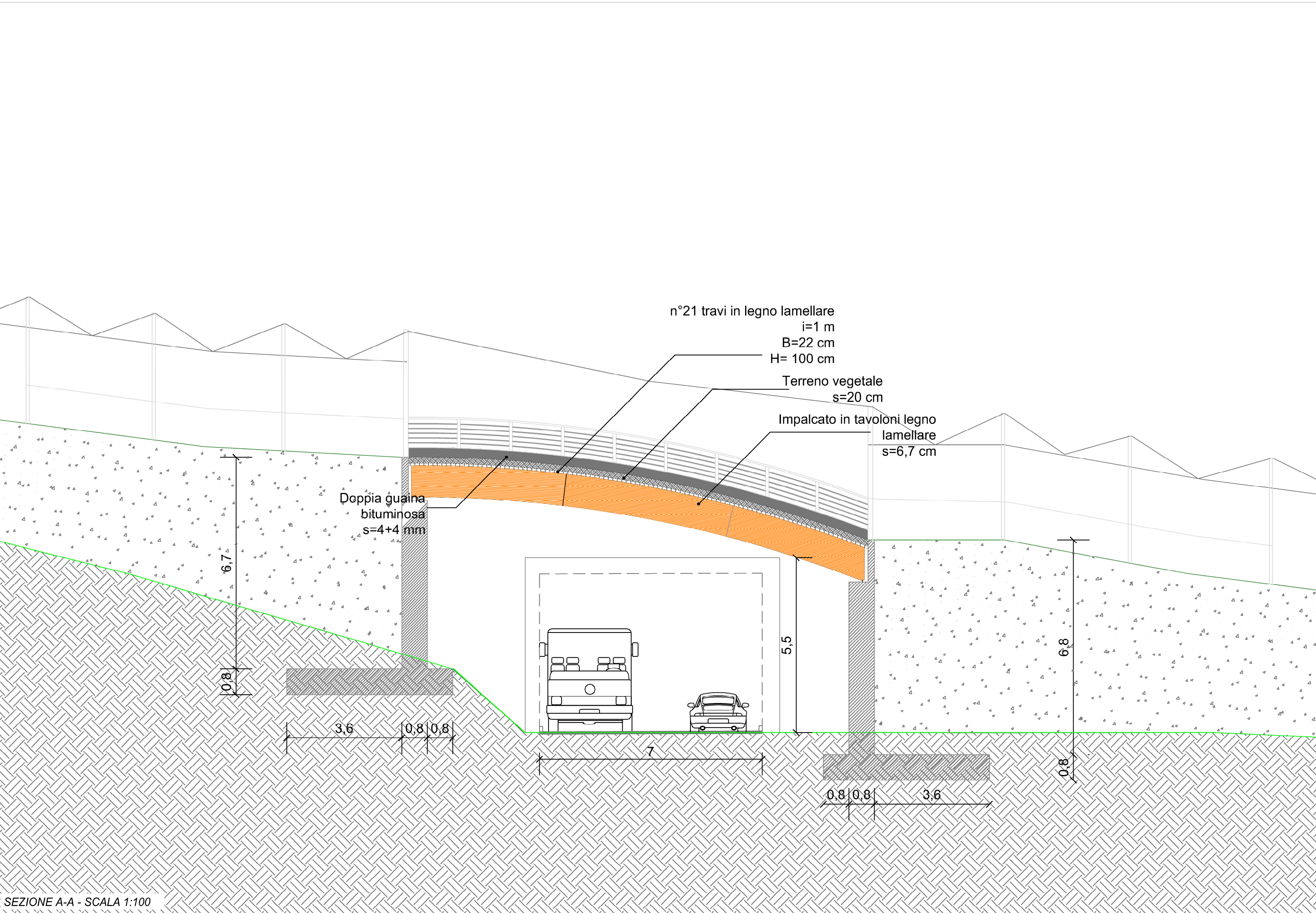
SEZIONE A-A - SCALA 1:100
