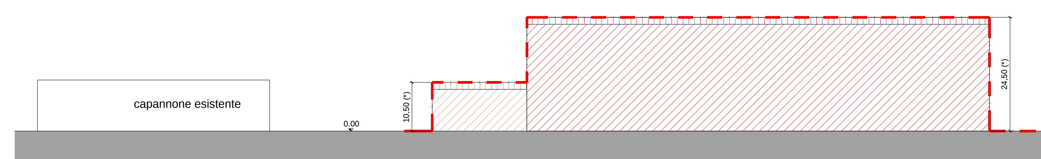
Sagoma limite lato est nuovo magazzino meccanizzato scala 1:500
