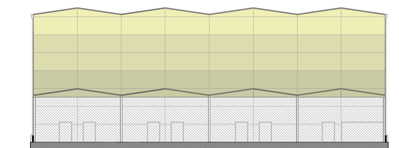
Prospetto sud scala 1:400
