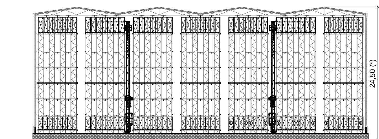
Sezione trasversale scala 1:400
