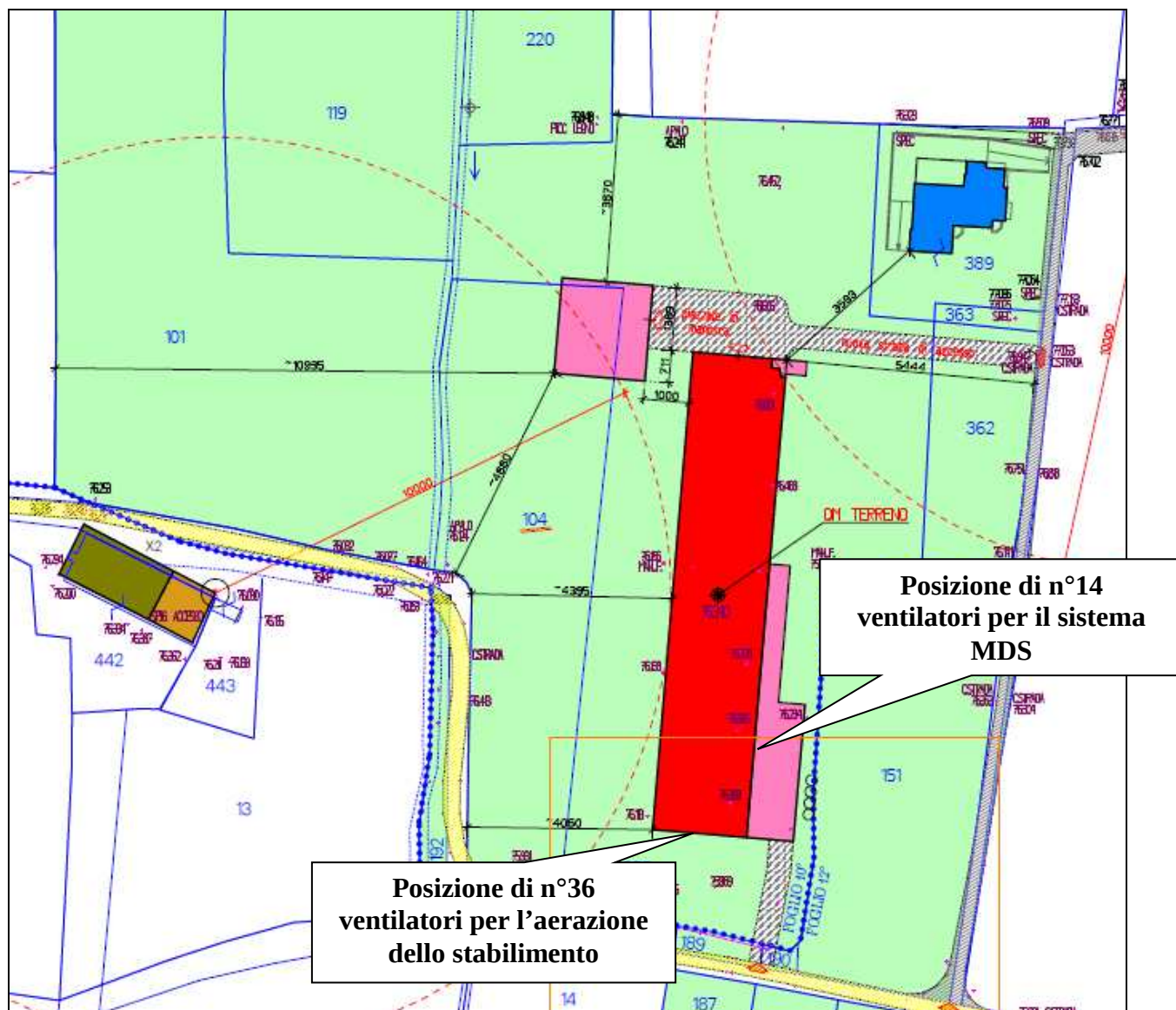
Fig. 2 : planimetria allo stato futuro segnalando la posizione delle sorgenti specifiche della Società
