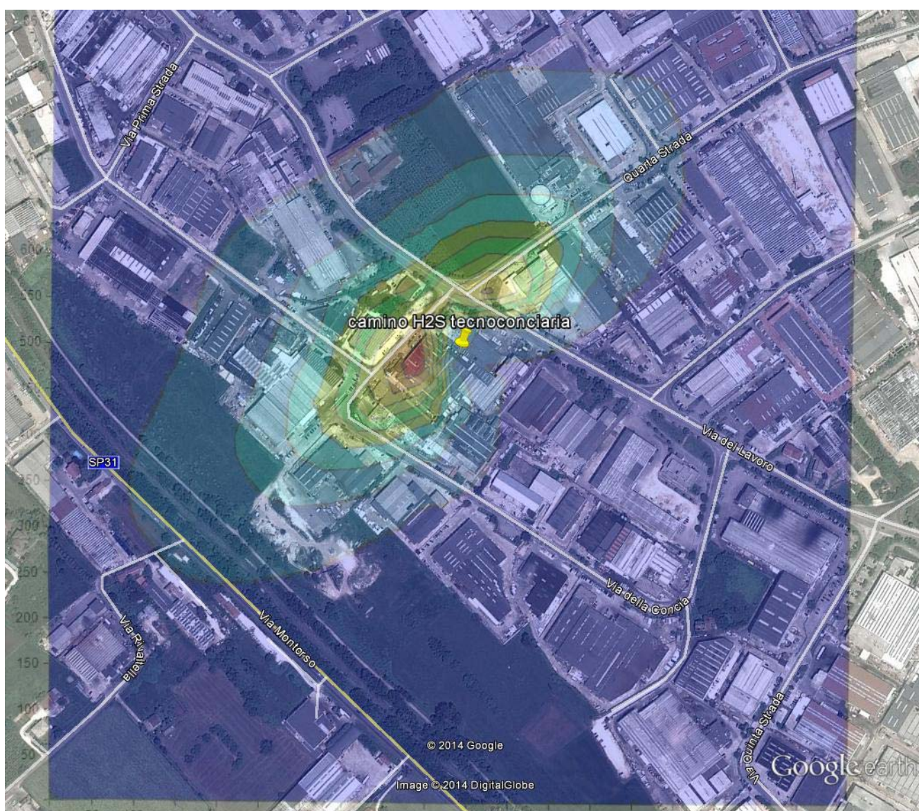
Figura 1 Valore medio annuale del livello totale di concentrazione di H2S espresso in \mu\text{g}/\text{m}^3
