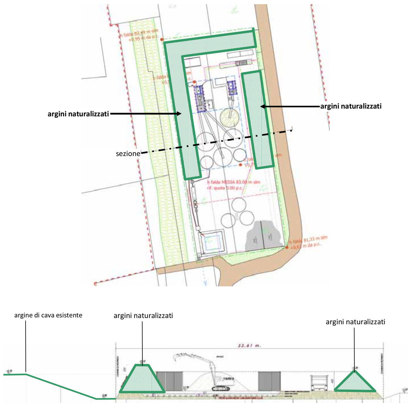
Figura 84: interventi di mitigazione di progetto.
