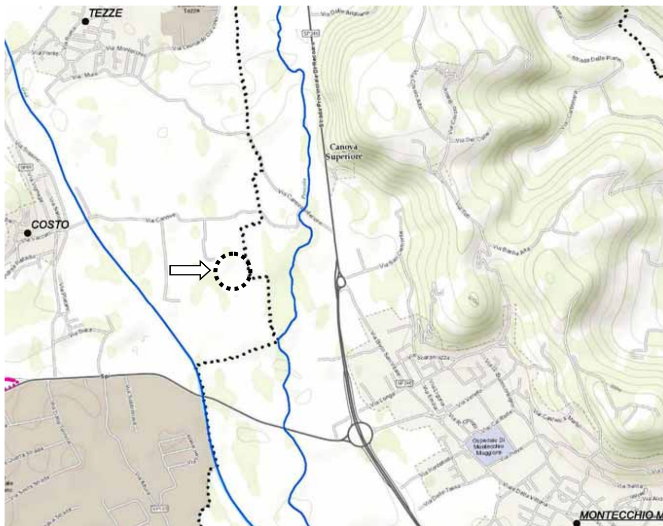
Figura 22: Aree allagabili, altezze idriche. Scenario di bassa probabilità (TR=300 anni).
