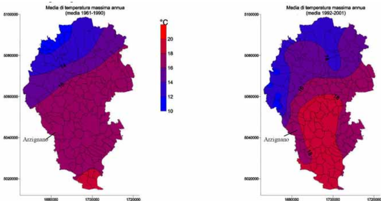
Figura 50: Distribuzioni dei valori medi annui della temperatura massima calcolati per il periodo di riferimento 1961-1990 e per il periodo 1992-2001 (fonte: VAS del PAT del Comune di Arzignano).
