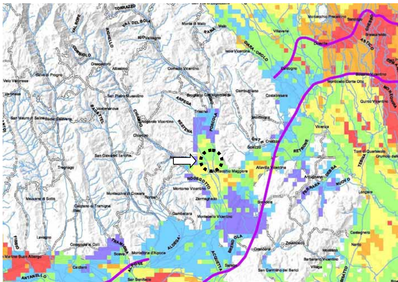
Figura 13: TAV. 2.2 Carta della vulnerabilità intrinseca della falda freatica della pianura veneta.
