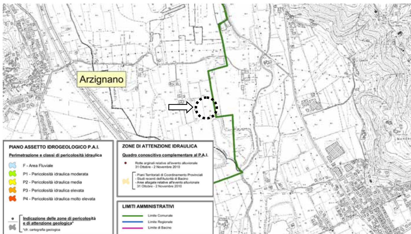
Figura 18: Piano di stralcio per l'Assetto Idrogeologico del bacino idrografico del fiume Brenta-Bacchiglione, Carta della pericolosità idraulica, Tavola 52, aggiornata con Decreto Segretariale n. 2432 del 25/09/2013.
