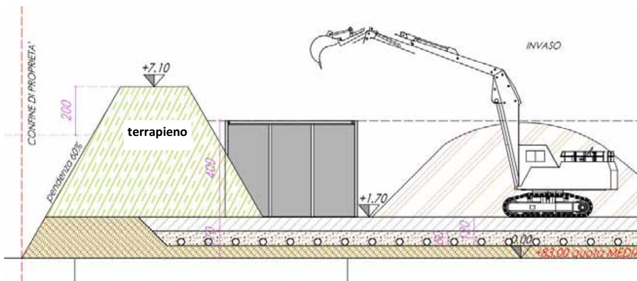
Figura 90: estratto sezione di progetto con particolare del terrapieno di contenimento delle emissioni acustiche.
