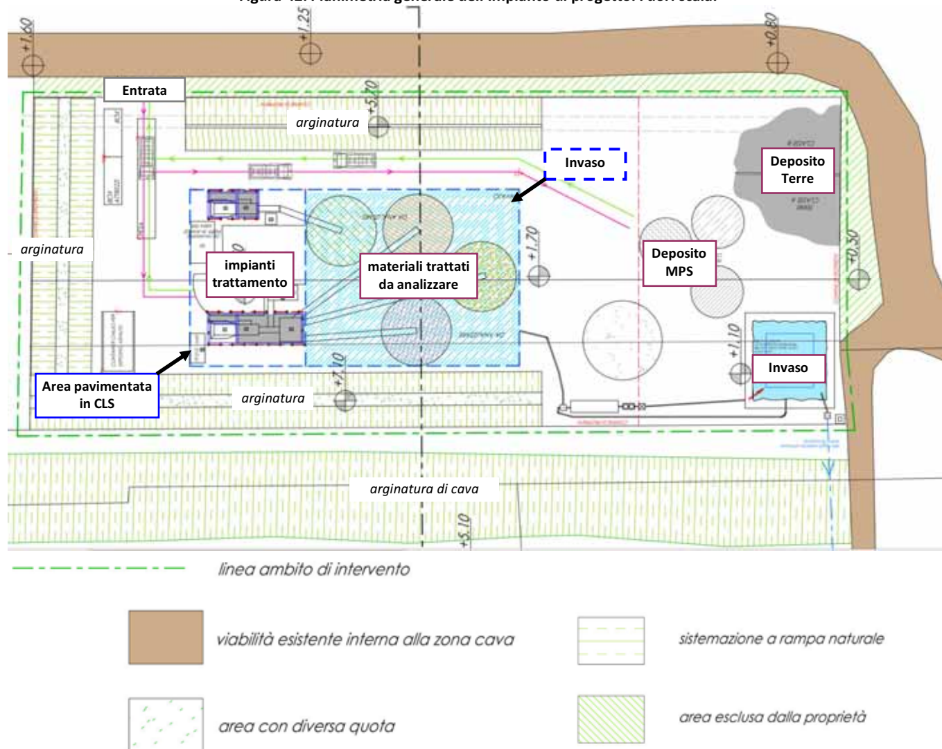
Figura 42: Planimetria generale dell'impianto di progetto. Fuori scala.
