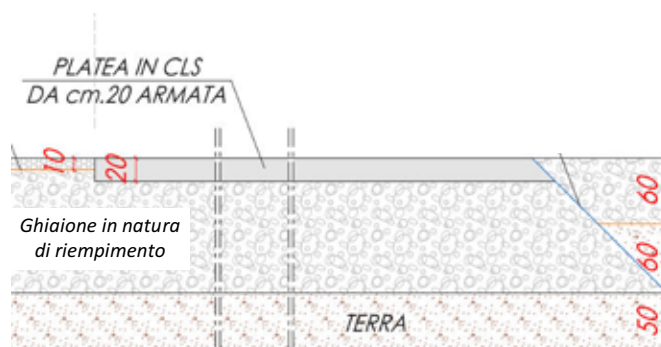
Figura 43: particolare dell'area impermeabilizzata per lo stoccaggio dei rifiuti inerti da trattare e degli impianti di lavorazione.
