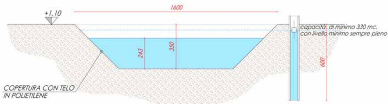
Figura 45: schema della vasca di accumulo delle acque di prima pioggia trattate e delle acque di seconda pioggia.
