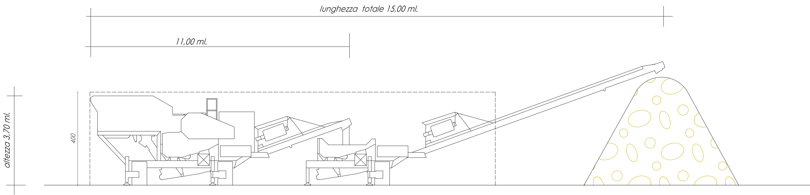
PROSPETTO TIPO IMPIANTO scala 1:100
