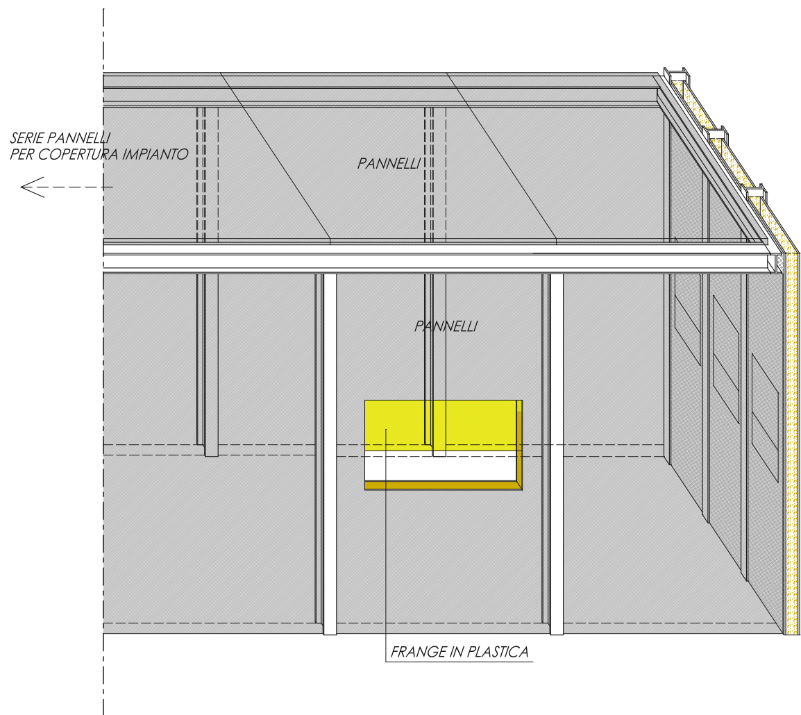
SEZIONE TIPO LATERALE MACCHINARIO USCITA NASTRO TRASPORTATORE
