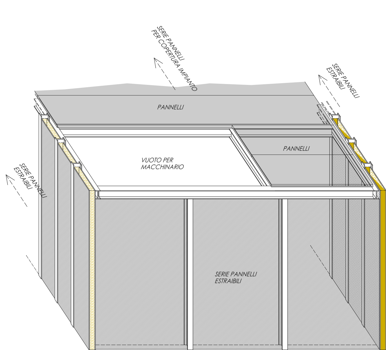
SEZIONE TIPO FRONTE MACCHINARIO
