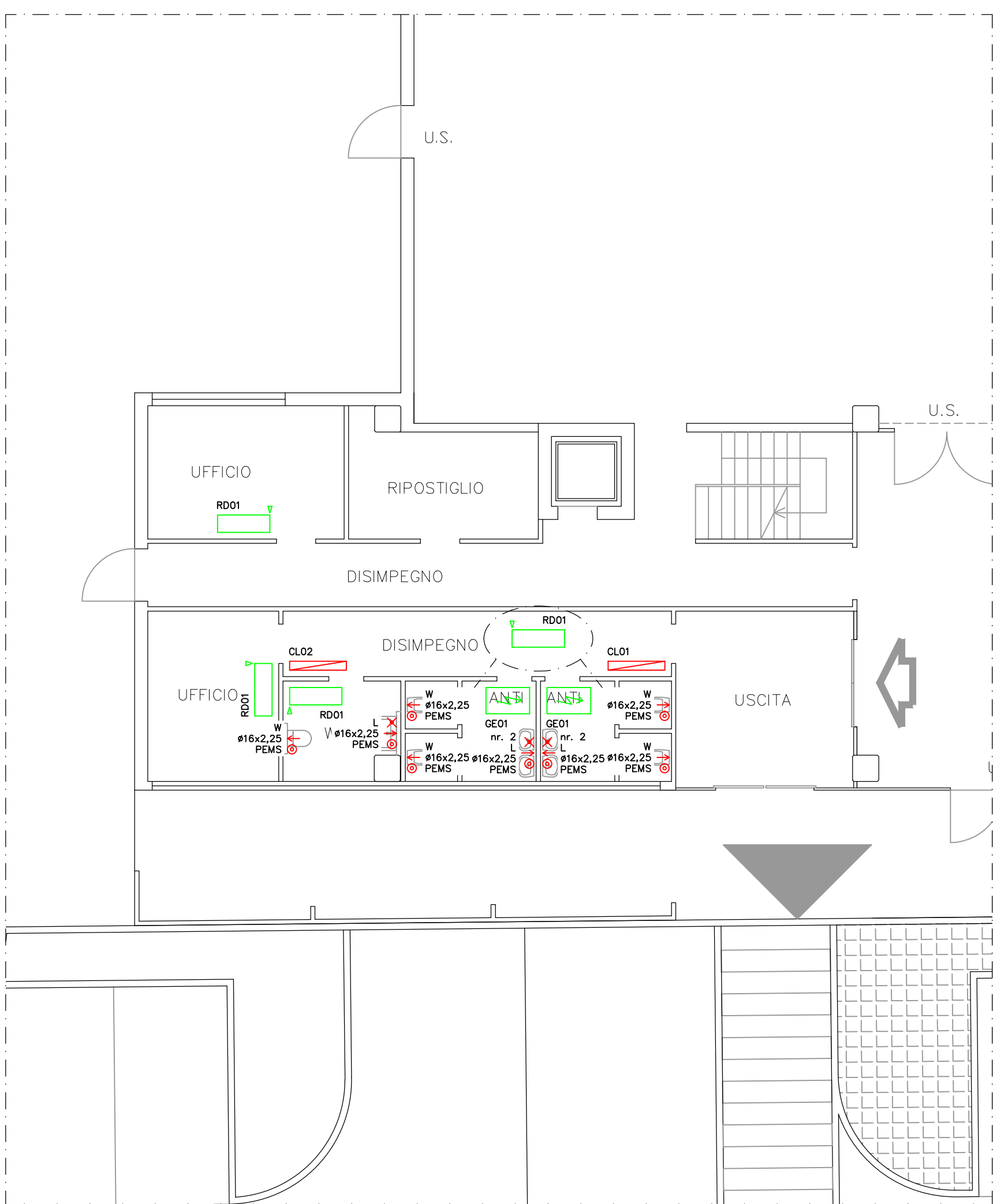
PIANTA PIANO TERRA – AREA SERVIZI/UFFICI 1
