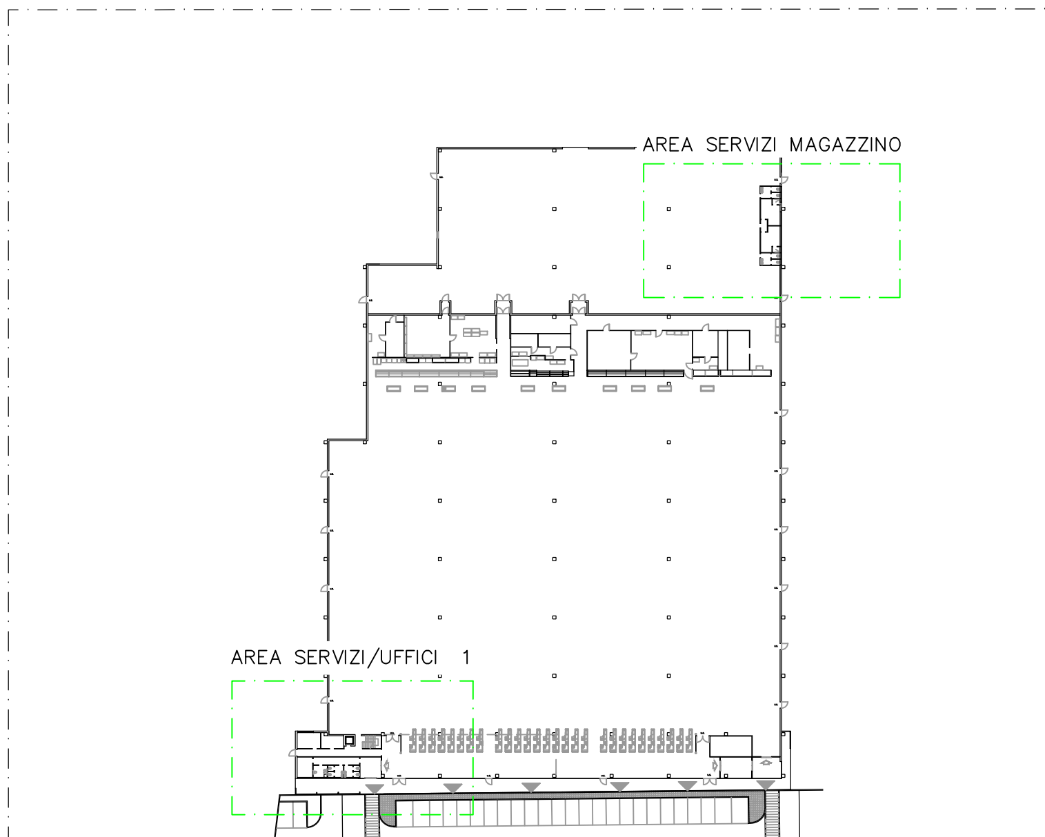
PIANTA PIANO TERRA – AREA SERVIZI MAGAZZINO
