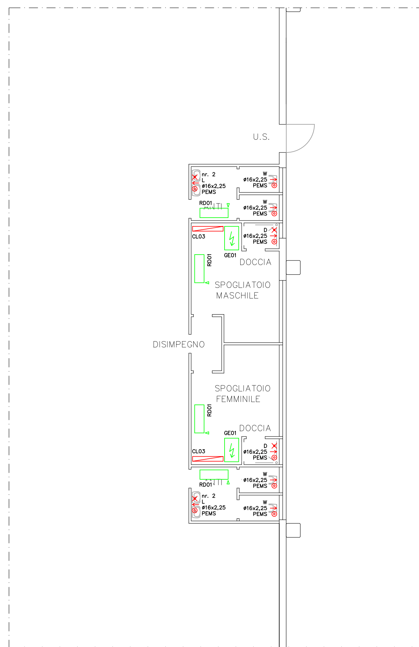
PIANTA PIANO TERRA – AREA SERVIZI MAGAZZINO
