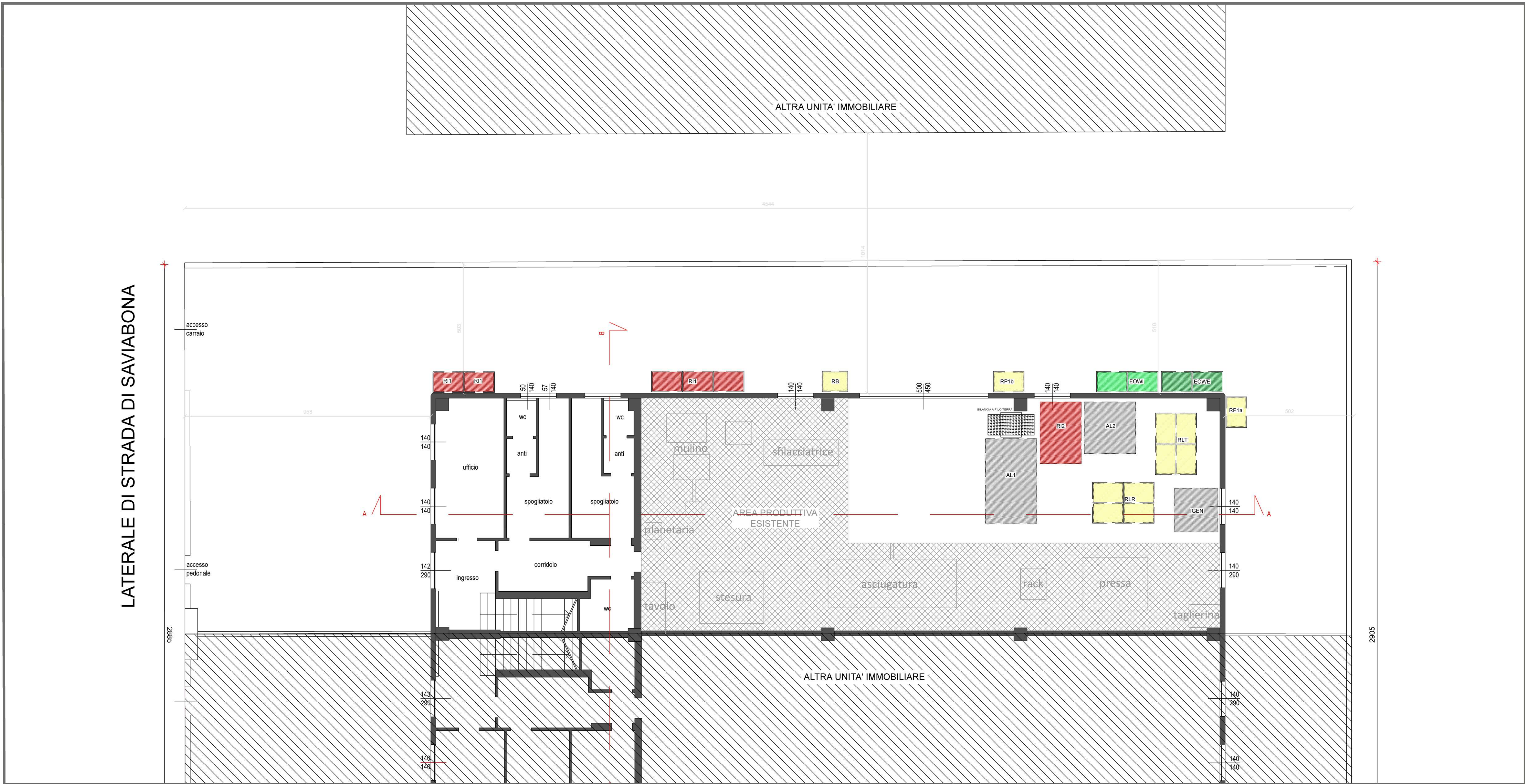
PIANTE - Stato di progetto - piano terra - scala 1 a 100
