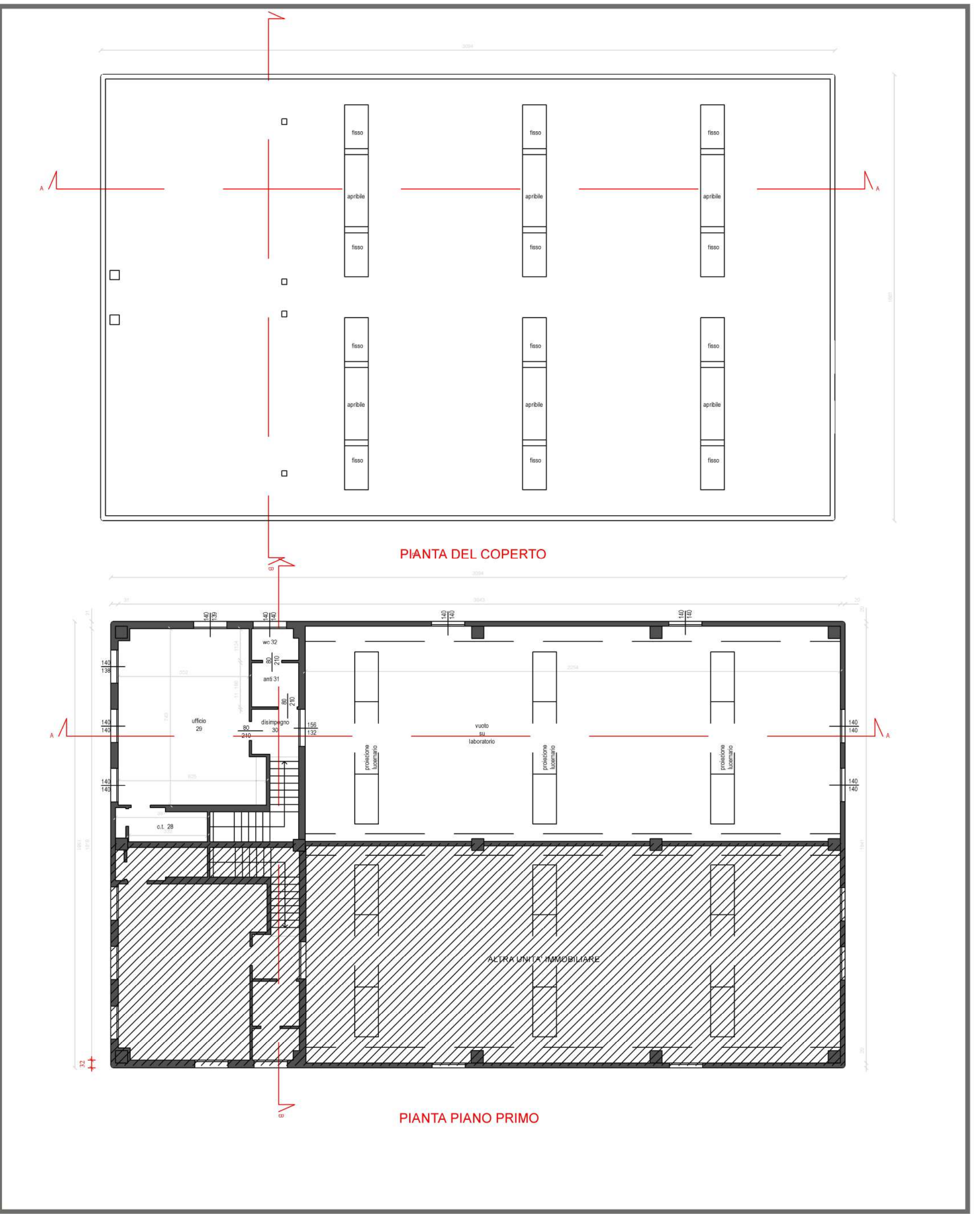
PIANTE - Stato di progetto - piano primo e copertura scala 1 a 200
