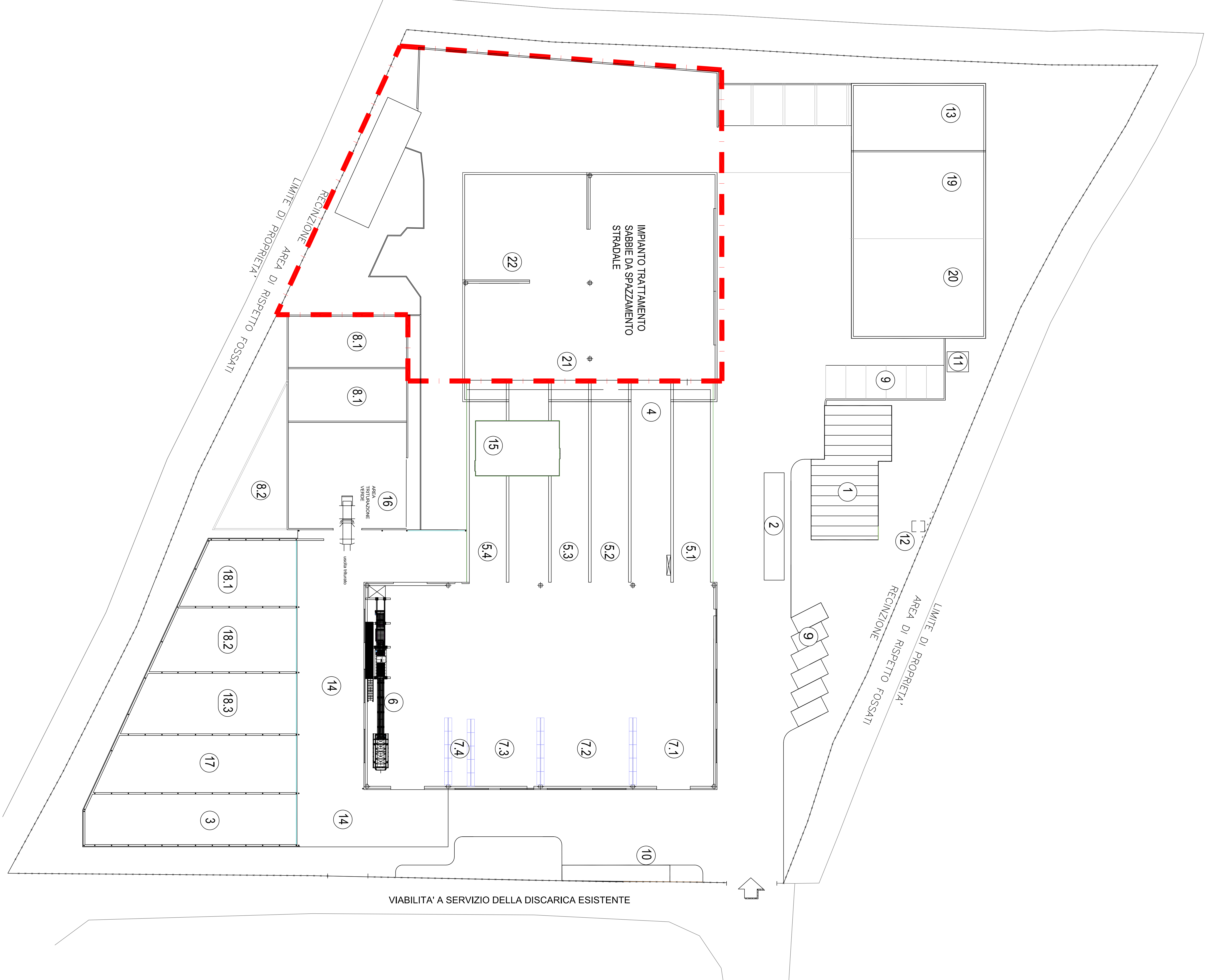
PLANIMETRIA GENERALE Scala 1:250
