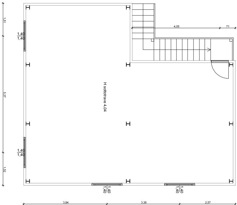
Planta Piano Primo uffici 1:100
