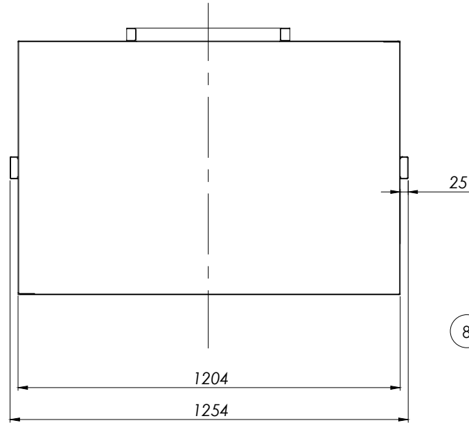
SEZIONE A-A
