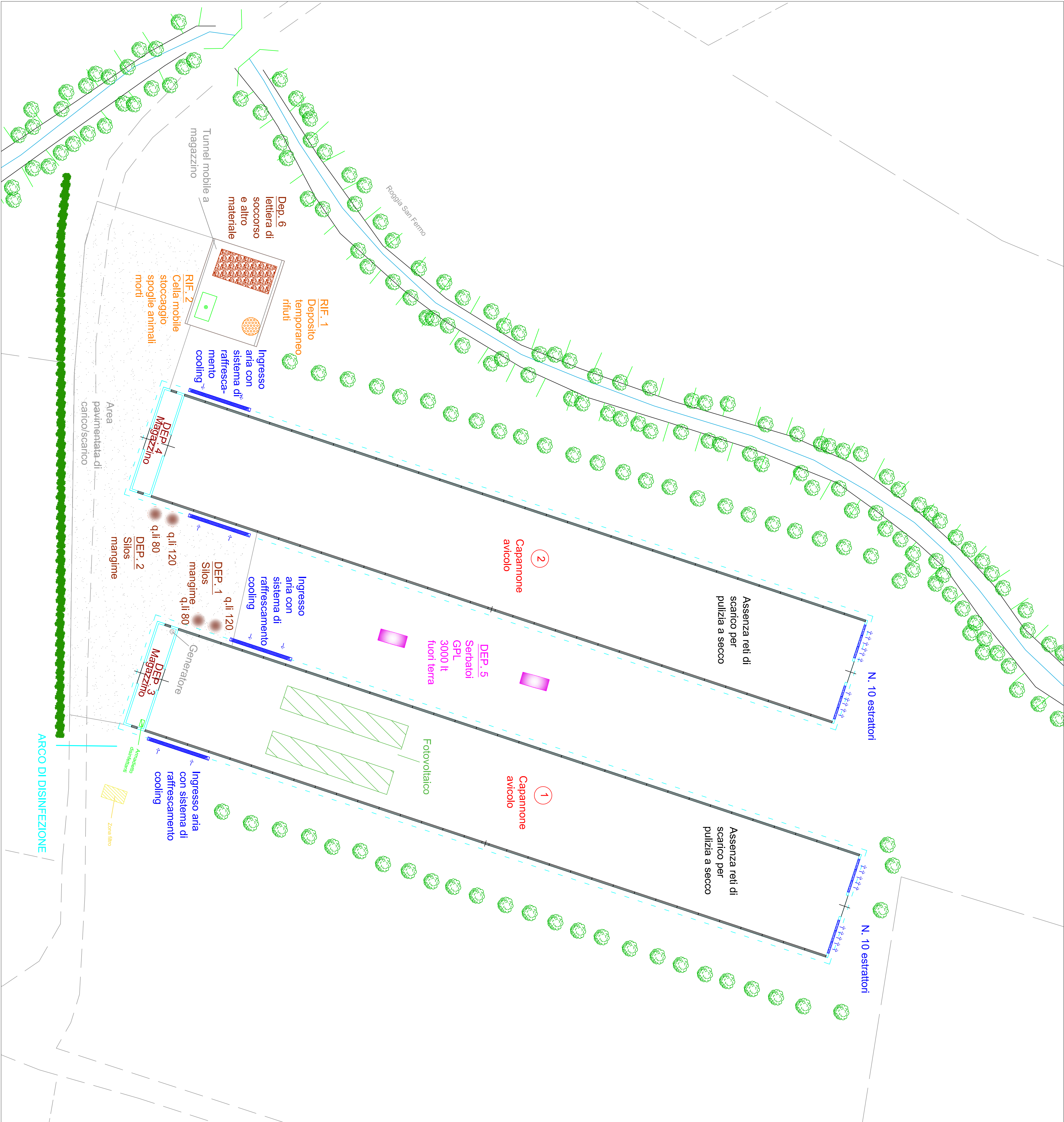
PLANIMETRIA GENERALE - Scala 1:400
