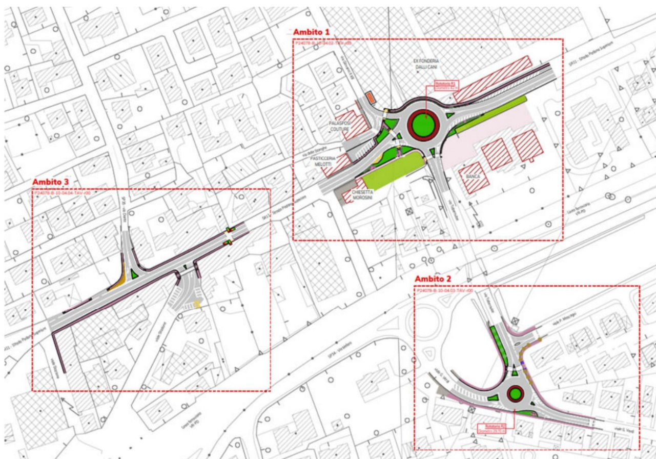
Figura 1: Planimetria generale di progetto
